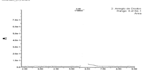
Figura 1a: Perfil de nifuratel (Ia) 1 mg/ml : 0,73 mg ln 0,73 ml de ACN Nifuratel (R) enanti
