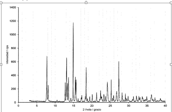
Figura 1: pXRD para la sal monohidrato cristalina de (S)-CSA de S-ketamina
