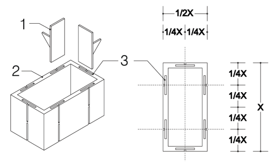
Isométrica mostrando módulos pasante (1), macetero (2) y orificios de conexión (3)
